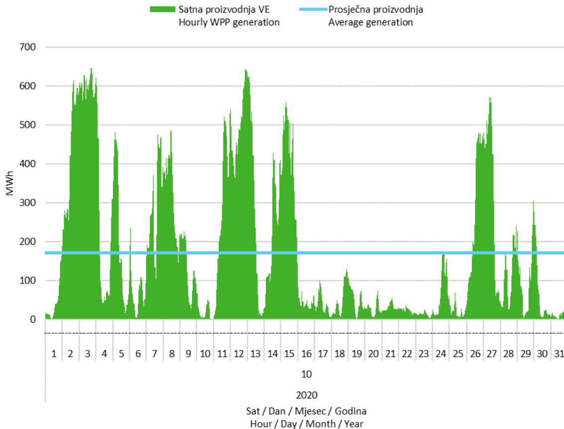
Slika 2 Satna proizvodnja svih vjetroelektrana u listopadu 2020. godine
