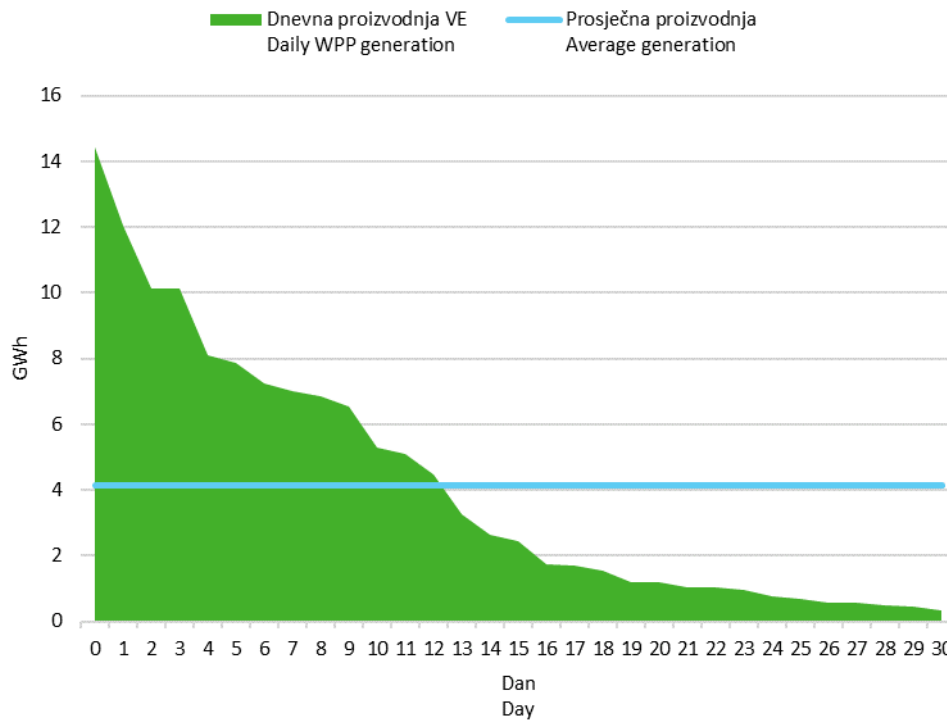
Slika 6 Krivulja trajanja dnevne proizvodnje vjetroelektrana u listopadu 2020. godine
