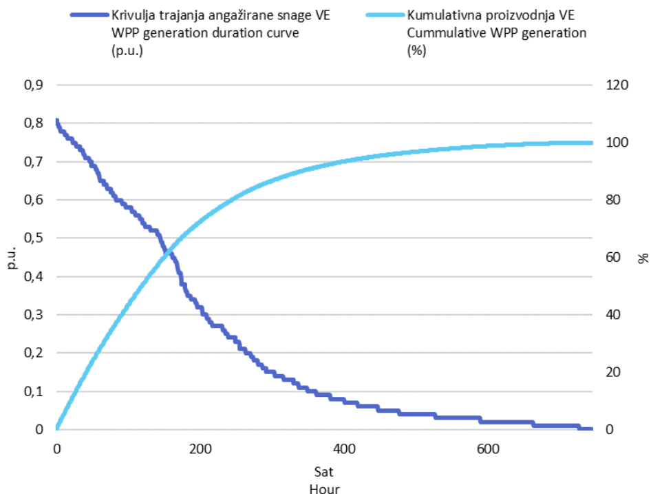
Slika 3 Krivulja trajanja angažirane snage svih VE i kumulativna proizvodnja VE u listopadu 2020. godine u jediničnim vrijednostima
