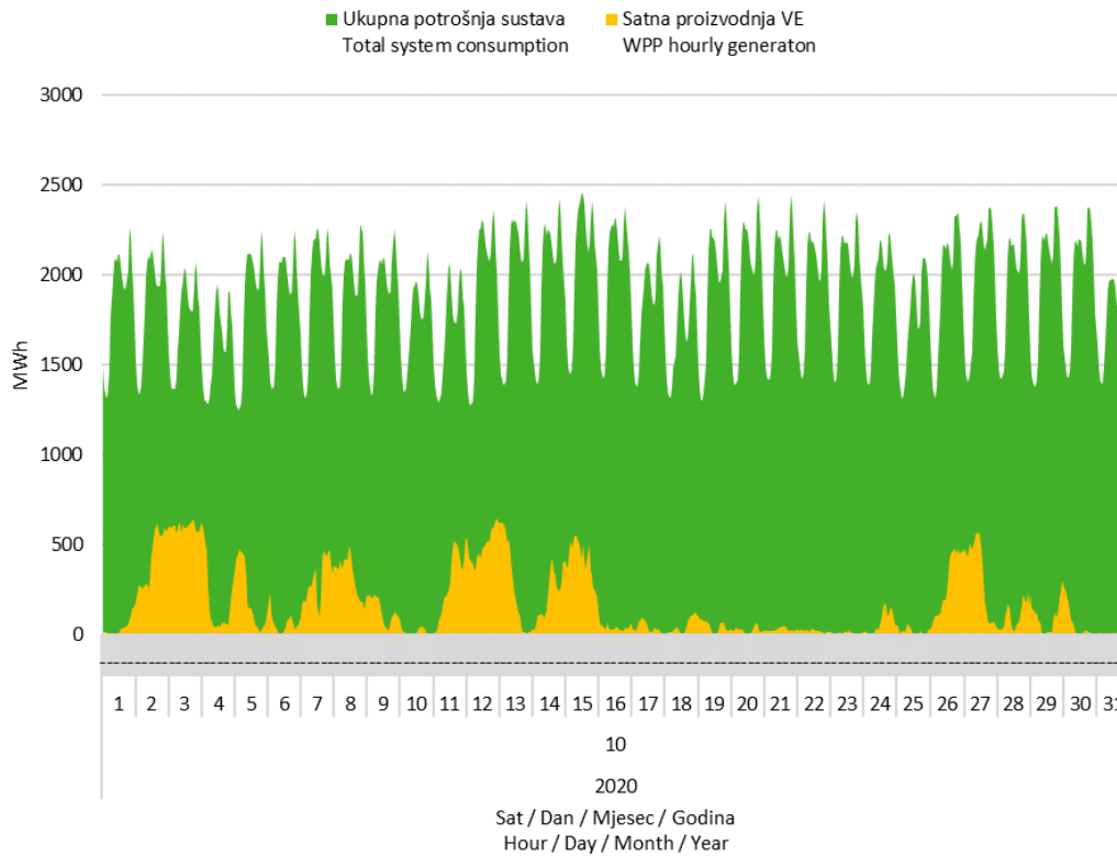
Slika 7 Usporedba satnog dijagrama opterećenja sustava i proizvodnje vjetroelektrana u listopadu 2020. godine
