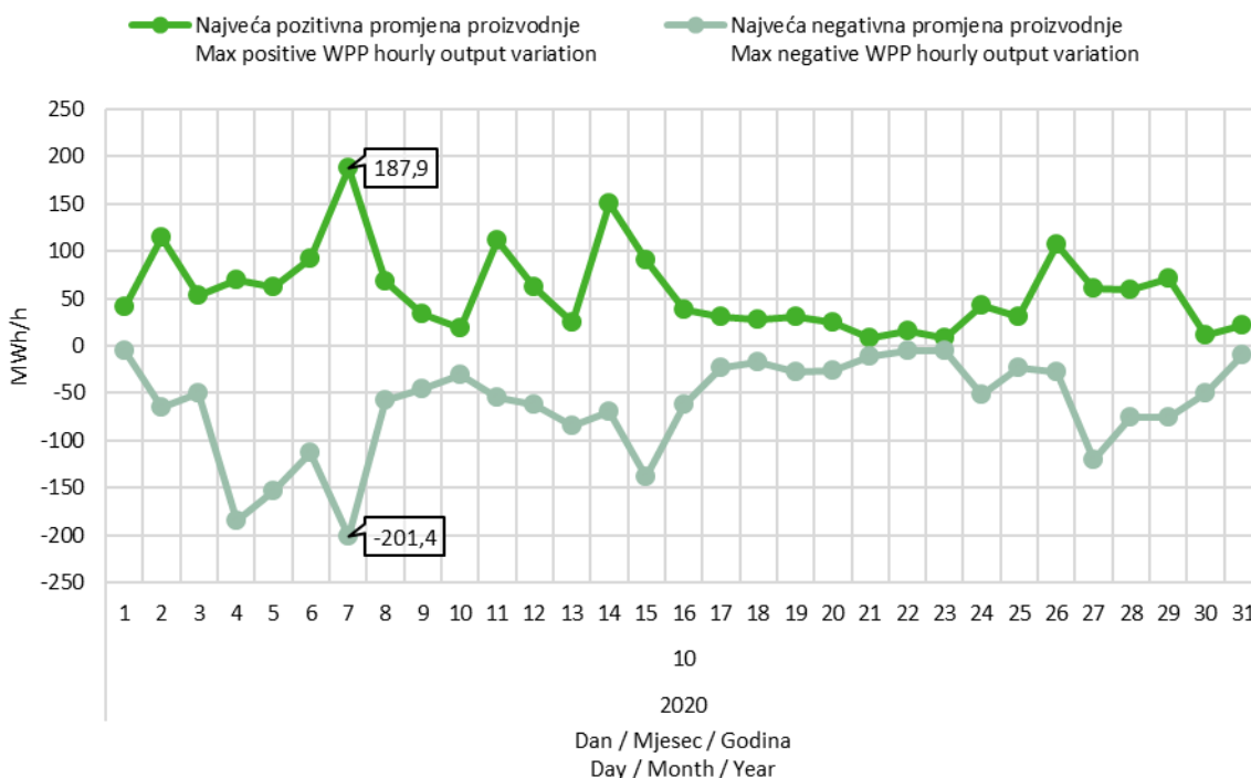
Slika 9 Maksimalna pozitivna i maksimalna negativna promjena satne proizvodnje VE u listopadu 2020. godine
