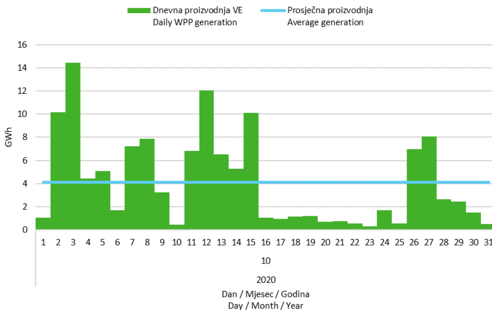
Slika 5 Dnevna proizvodnja svih vjetroelektrana u listopadu 2020. godine Figure 5 Daily generation of all wind power plants in October 2020
