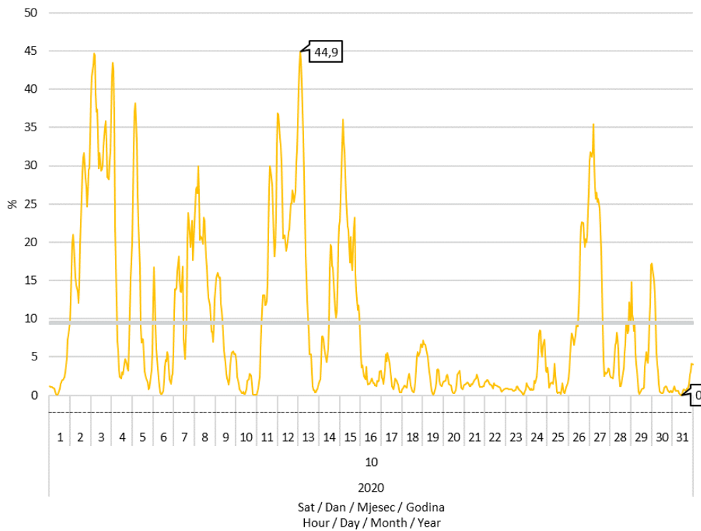
Slika 8 Udio proizvodnje vjetroelektrana u pokrivanju satnog opterećenja elektroenergetskog sustava u listopadu 2020. godine
